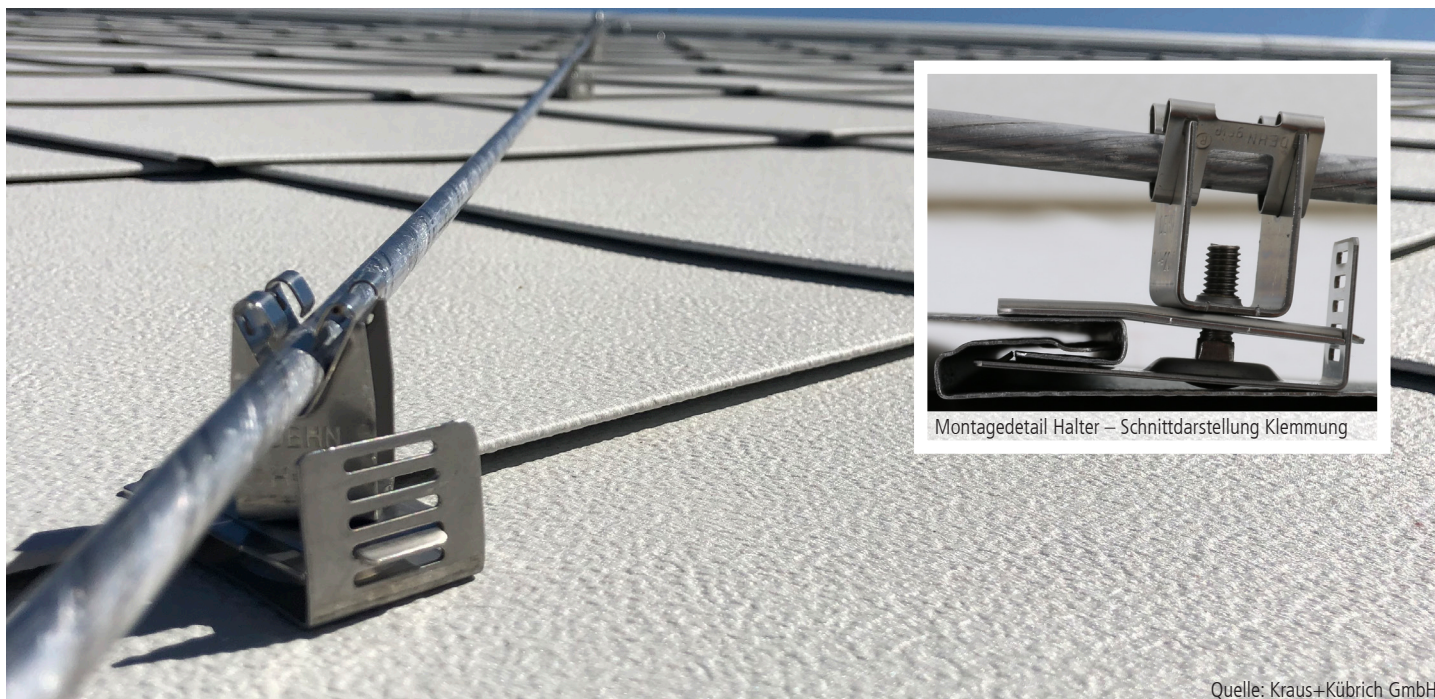
Dachleitungshalter auf PREFA Kleinformat Schindeln
