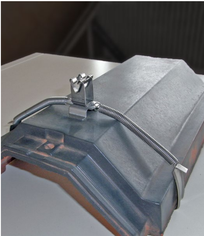
Erweiterung der Spannweite des Firstleitungshalters SPANNgrip.
