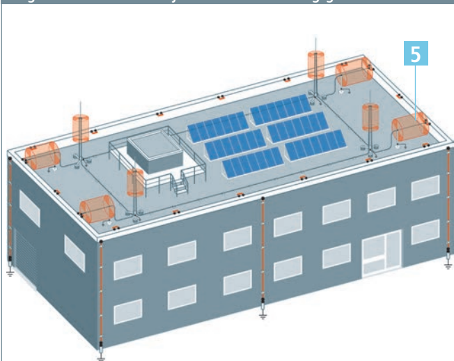
Getrenntes Blitzschutzsystem eines Verwaltungsgebäudes
