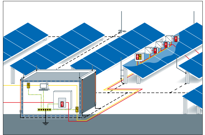
Solarpark mit Stringwechselrichter
