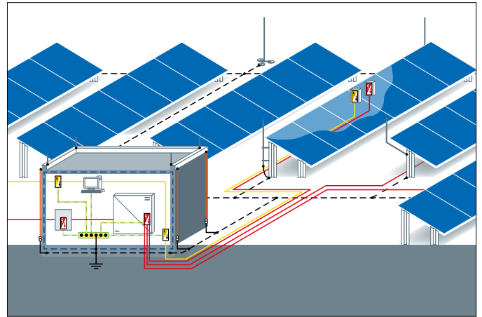
Solarpark mit Zentralwechselrichter
