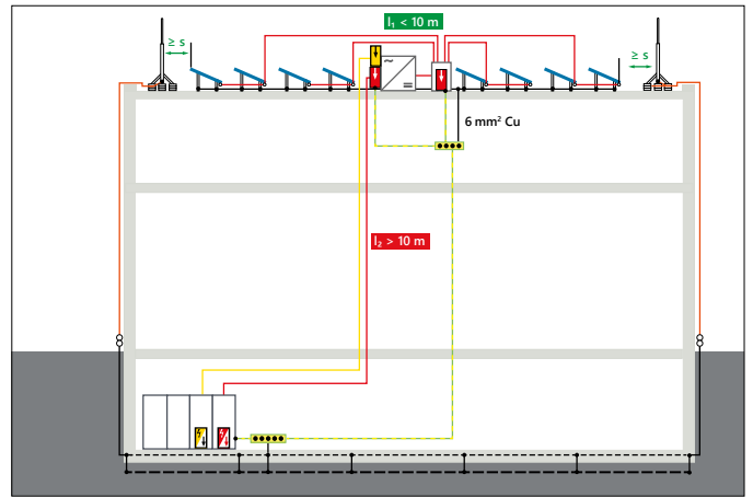
Gebäude mit konventionellem Blitzschutz: Trennungsabstand eingehalten
