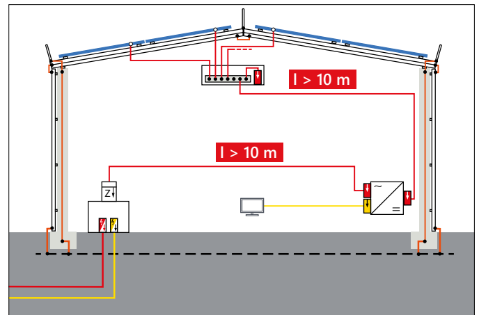
Gebäude mit äußerem Blitzschutzsystem: Metалldach
