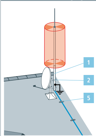
Wohnhaus / Aufdachverlegung
