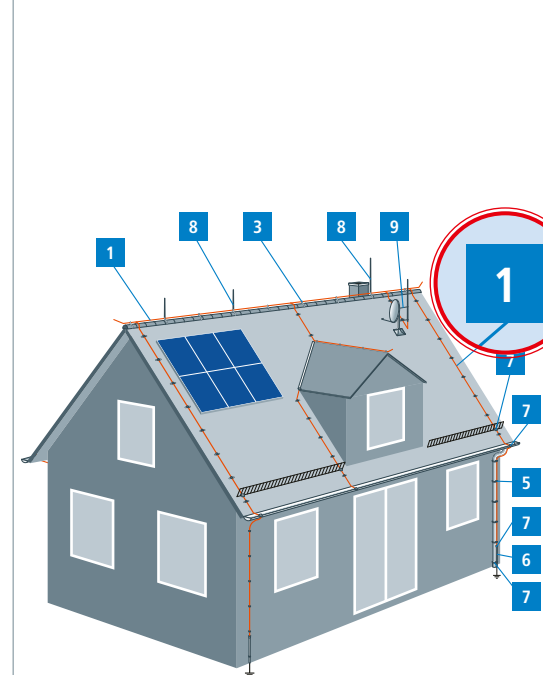
Äußerer Blitzschutz eines Wohnhauses
