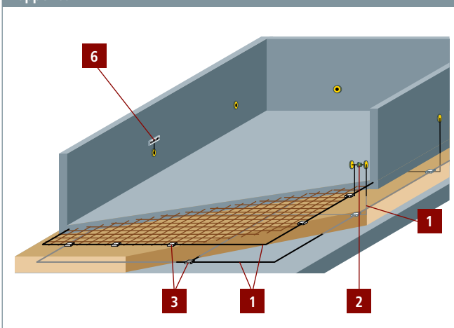
Fundamenterder nach OVE E 8014 ohne Blitzschutzsystem; stahlbetonbewehrte Bodenplatte, kein WU-Beton oder keine Vollperimeterdämmung, Noppenbahn oder ähnliches.
