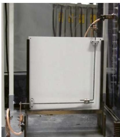
Bild 5: Auf Isolierplatte befestigter Prüfling (MV-Klemme) für Test im Stoßstromlabor.
