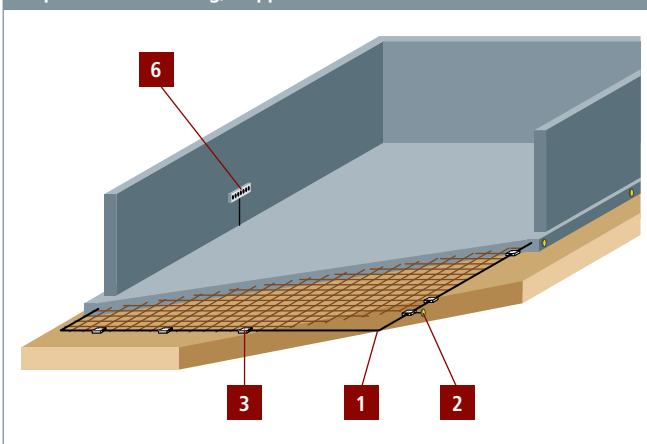
Fundamenterder nach OVE E 8014 ohne Blitzschutzsystem; stahlbetonbewehrte Bodenplatte, kein WU-Beton oder keine Vollperimeterdämmung, Noppenbahn oder ähnliches.
