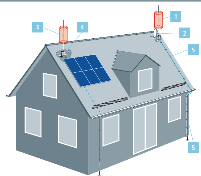
Wohnhaus / Unterdachverlegung
