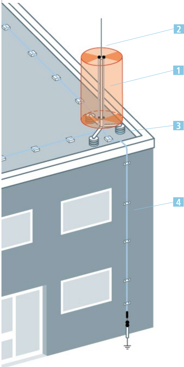
Getrenntes Blitzschutzsystem eines Verwaltungsgebäudes
