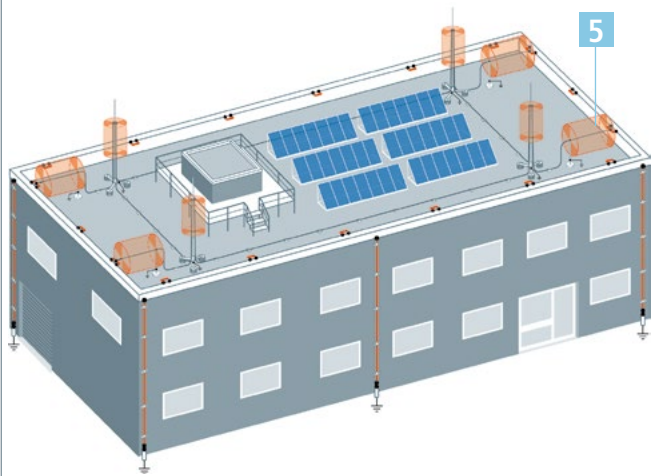
Getrenntes Blitzschutzsystem eines Verwaltungsgebäudes
