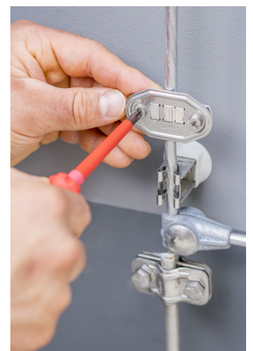
4. Schritt: Das fertig bestückte Nummernschild wird an der Ableitung befestigt.
